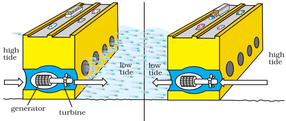
Fig. 3.22: Tidal Energy
